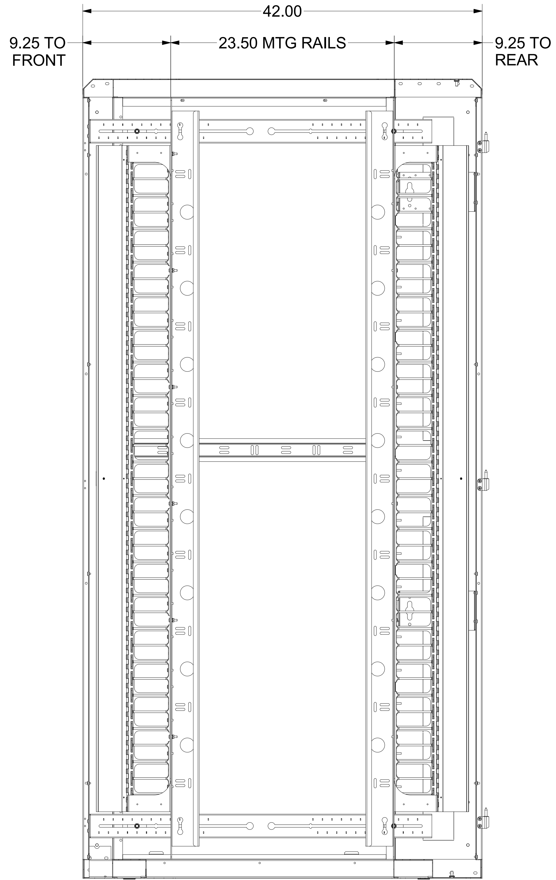
SECTION A-A
