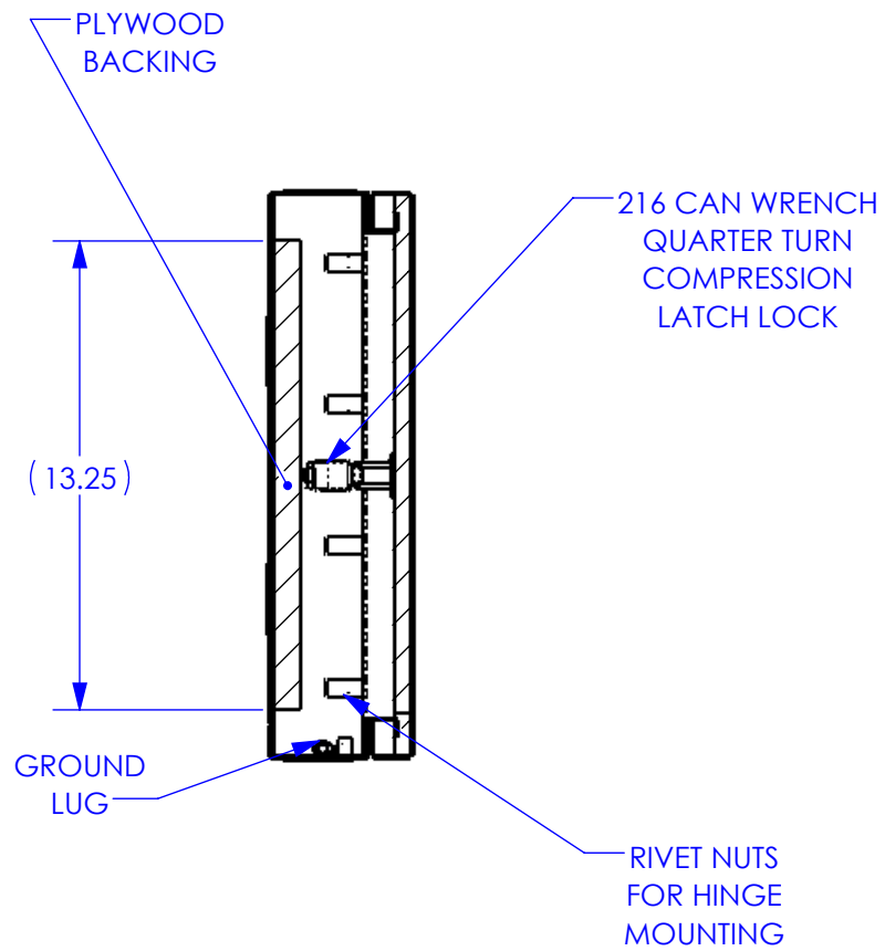
SECTION B-B SCALE 1 : 6
