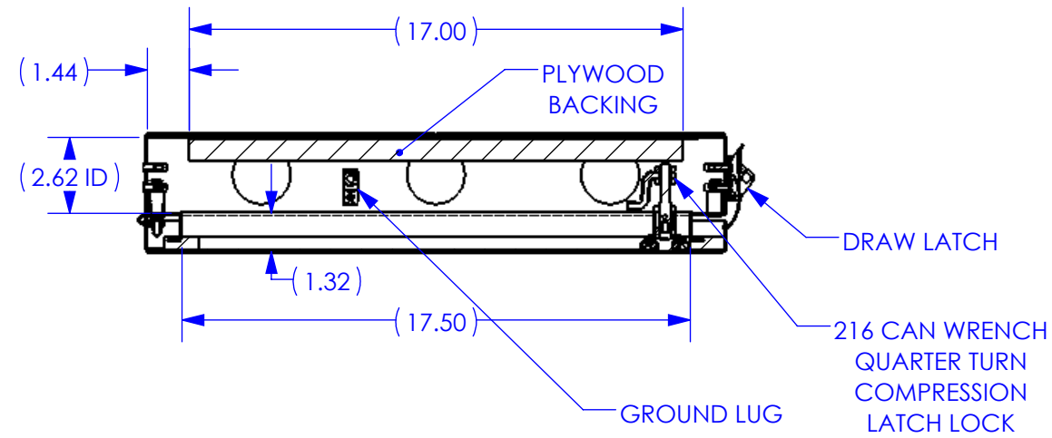
SECTION A-A SCALE 1 : 6
