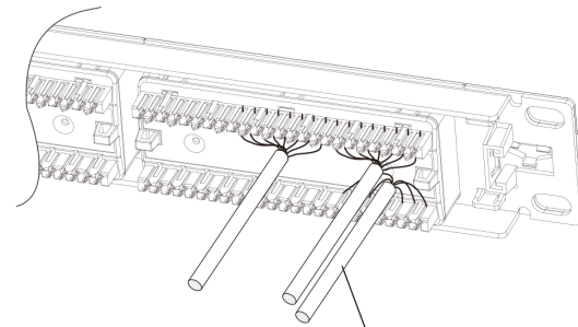
Solid Cable
